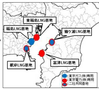
東京湾内のLNG基地
